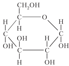
Фруктоза
