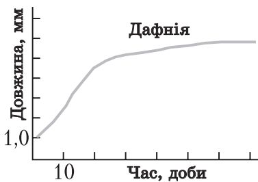
Обмежений ріст
