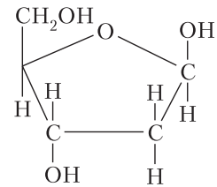
Дезоксирибоза
