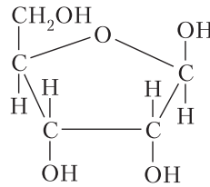
Рибоза
