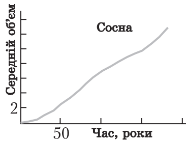
Необмежений ріст
