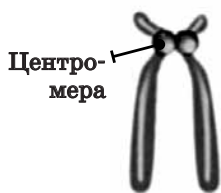
Телоцентрична хромосома
