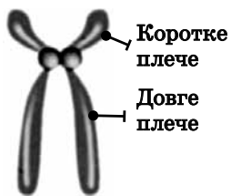
Акроцентрична хромосома
