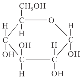
Глюкоза
