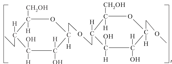
Целюлоза
