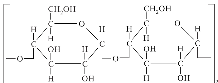
Крохмаль
