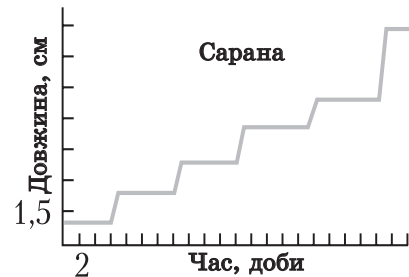
Періодичний ріст
