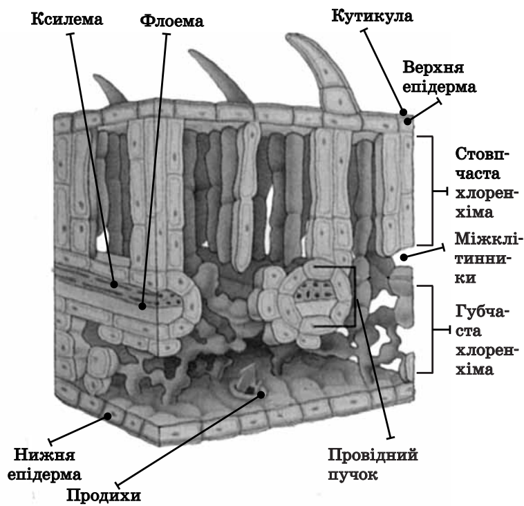
Будова листка
